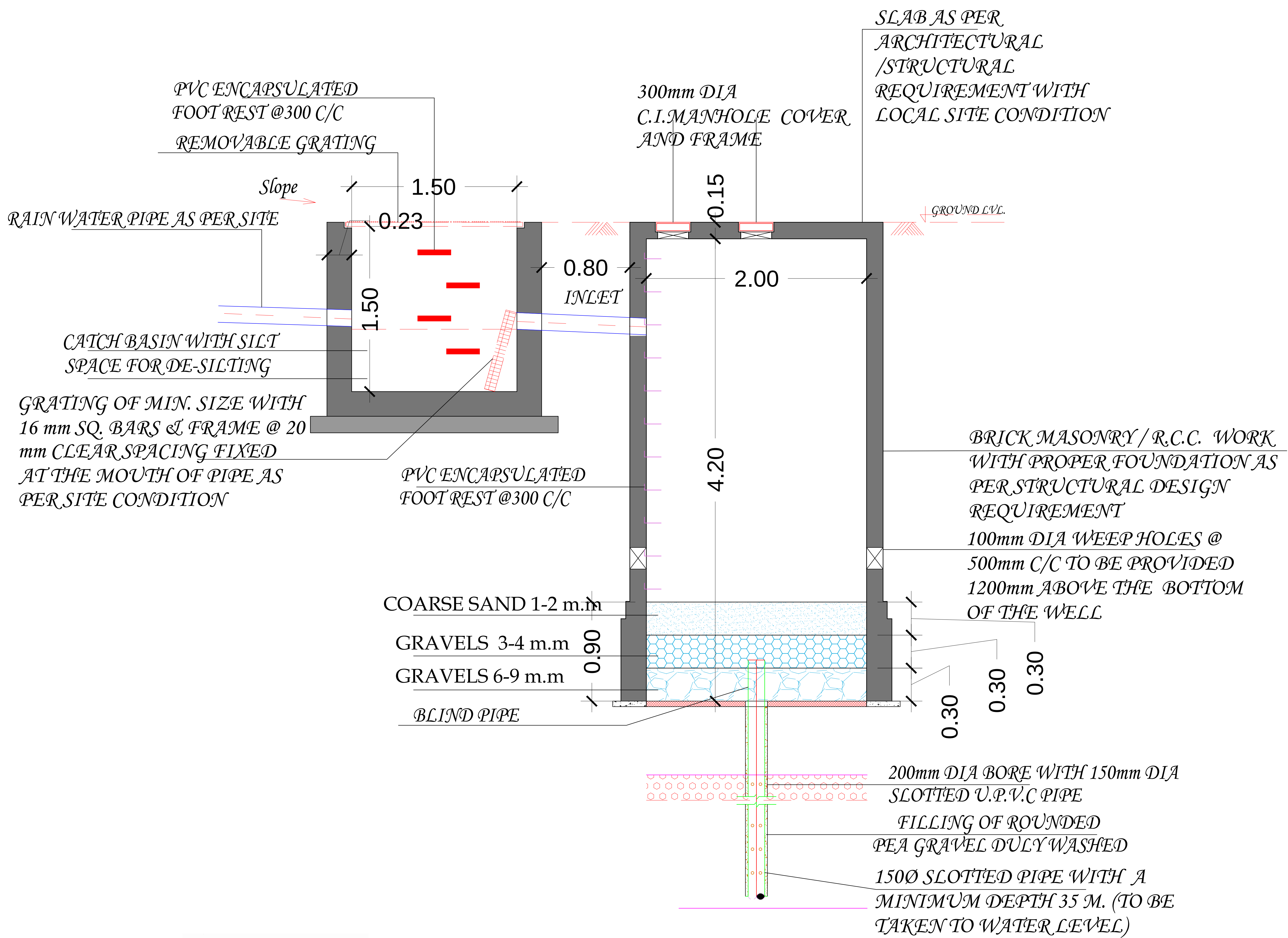
SECTION A-A
